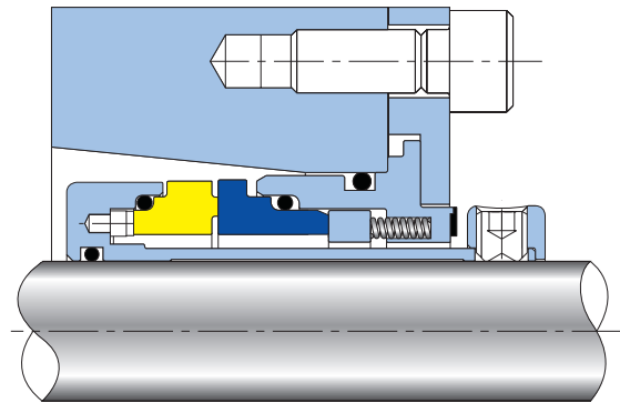
AESSEAL® MOGCE™
