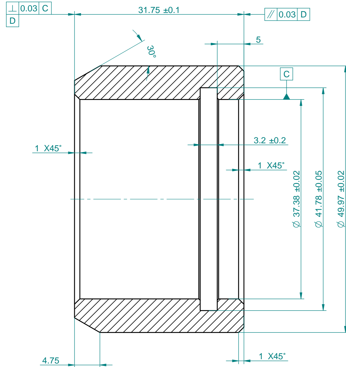
SECTION A-A
